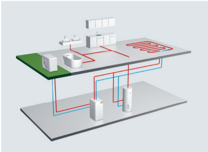
Schematische Darstellung von Raumheizung und Warmwasseraufbereitung bei einem Einfamilienhaus mit der Luft-Wasser-Wärmepumpe Bosch CS5800i AW 7 ORE-S.
